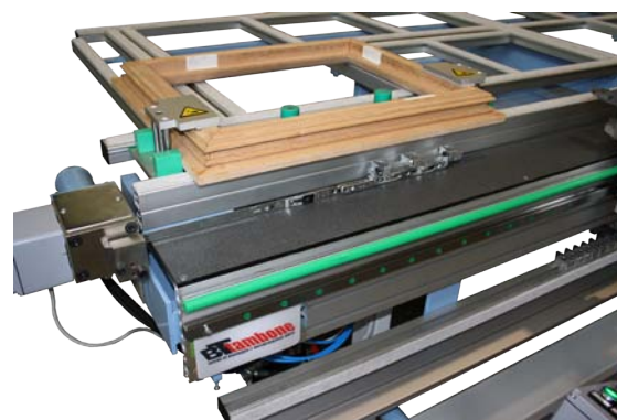
Rilevamento automatico della misura di taglio Automatic reading of cut measurement
